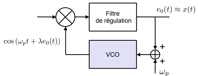
Démodulateur FM: Phase-Locked Loop (PLL)
